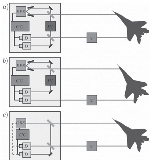
Obrázek č. 4: Tři návrhy kvantových radarů: a) kvantová interference, b) kvantová iluminace, c) kvantové homodynní měření. Tmavě modré obdélníky představují zrcadla, světle modré obdélníky představují polopropustná zrcadla, červená čára reprezentuje šíření fotonů a jednotlivé součásti jsou: EPS - zdroj kvantově provázaných fotonů, CRS - zdroj koherentních fotonů, PI - zdržení, zpoždění druhého drženého fotonu, D - detektor, CC - řídicí počítač a \varphi je fázové zpoždění, reprezentující cestu k cíli a zpět.
